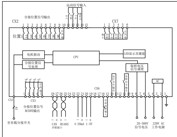
YK-4A接线图（适用于 N \leq 9 ）
