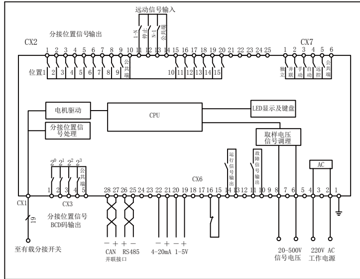
YK-4A 接线图 (适用于 N \leq 15 )
