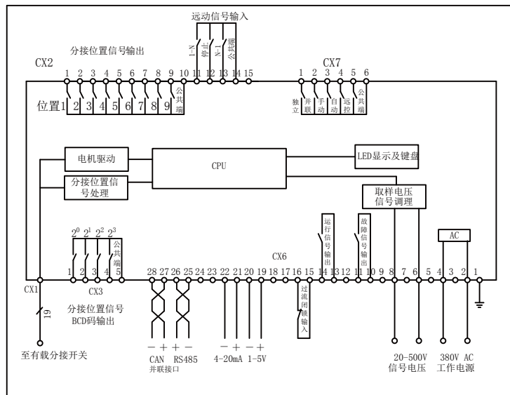
YK-3A 接线图（适用于 N \leq 9 ）
