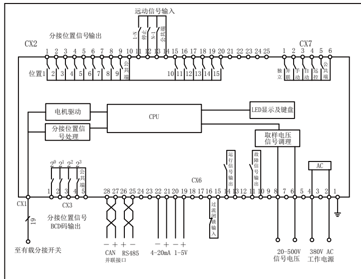
YK-3A 接线图 (适用于 N \leq 15 )
